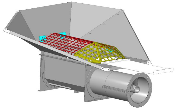
Trichter 6-eckig RGK 200
