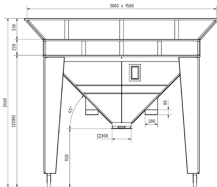
Maßzeichnung
