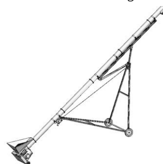
Fahrgestell
